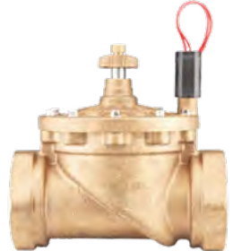
IBV-301G-FS Diámetro de entrada: 3" (80 mm) Altura: 23 cm Longitud: 22 cm Anchura: 18 cm
