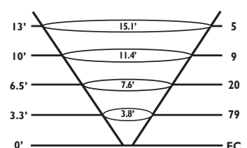
MR-16 50W 60°
