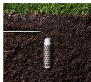
Sonde Soil-Click™
